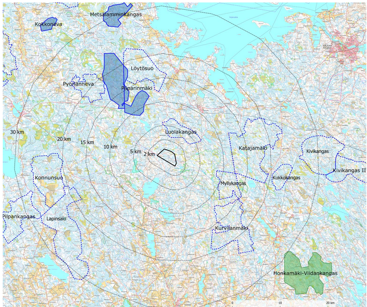
Kuva 7. Rakennetut tuulivoimapaistot sekä hyväksytyt ja vireillä olevat tuulivoimahankkeet suunnittelualueen ympäristössä. Metsälamminkankaan, Kokkonevan ja Piiparinmäen tuulivoimapaistot ovat tuotannossa (siniharmaat alueet). Honkamäki-Viidankankaan hankkeen kaava on hyväksytty (vihreä alue). Muissa hankkeissa YVA-menettelyt ja kaavoitus ovat käynnissä (tilanne 7.7.2025).
