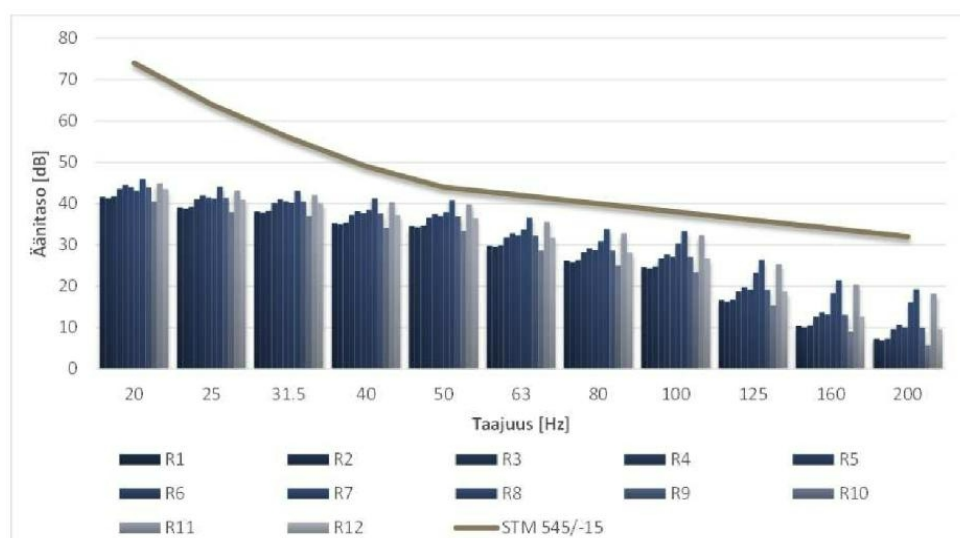
Kuva 8-18. Pientaajuisten melulaskennan tulokset (vastaa YVA-menettelyssä tutkittua hankevaihtoehtoa VE1).
