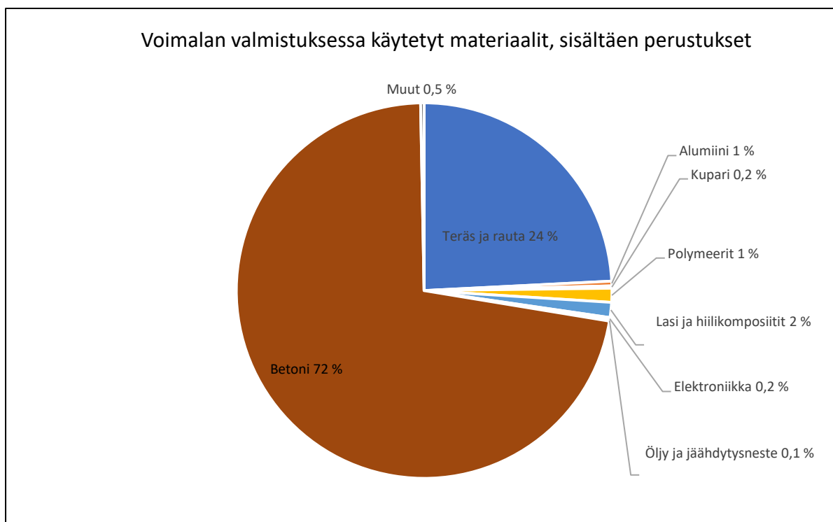
Kuva 8-22. Esimerkki voimalan valmistuksessa käytettävistä materiaaleista sisältäen voimalaperustukset, ja niiden osuus koko voimalan massasta (mukaillen Vestas 2023).
