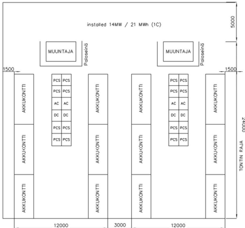
Kuva 2-8. Periaatekuva energiavarastosta.
