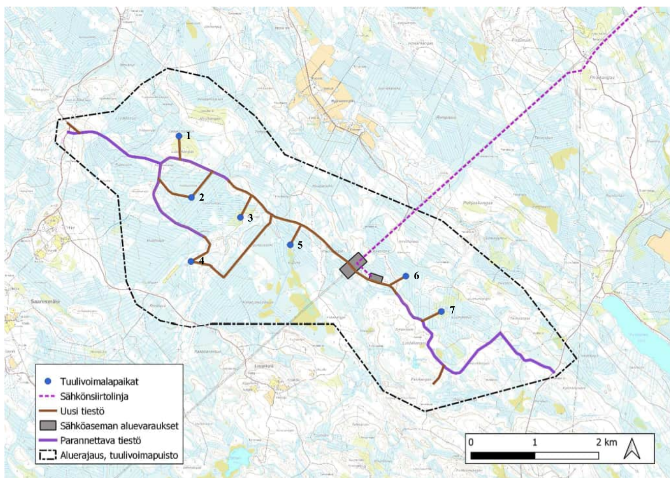
Kuva 1. Luolakan tuulivoimapuiston aluerajaus, tiestö, tuulivoimaloiden suunnitellut sijoituspaikat (7 kpl) ja sähkönsiirtoon tarkoitettun voimajohtohankkeen (SVE2) suunniteltu linjaus.
