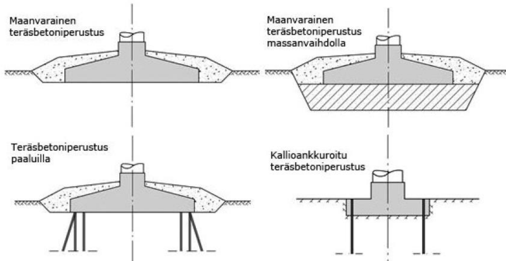
Kuva 2-4. Tuulivoimaloiden perustamistekniikoita.
