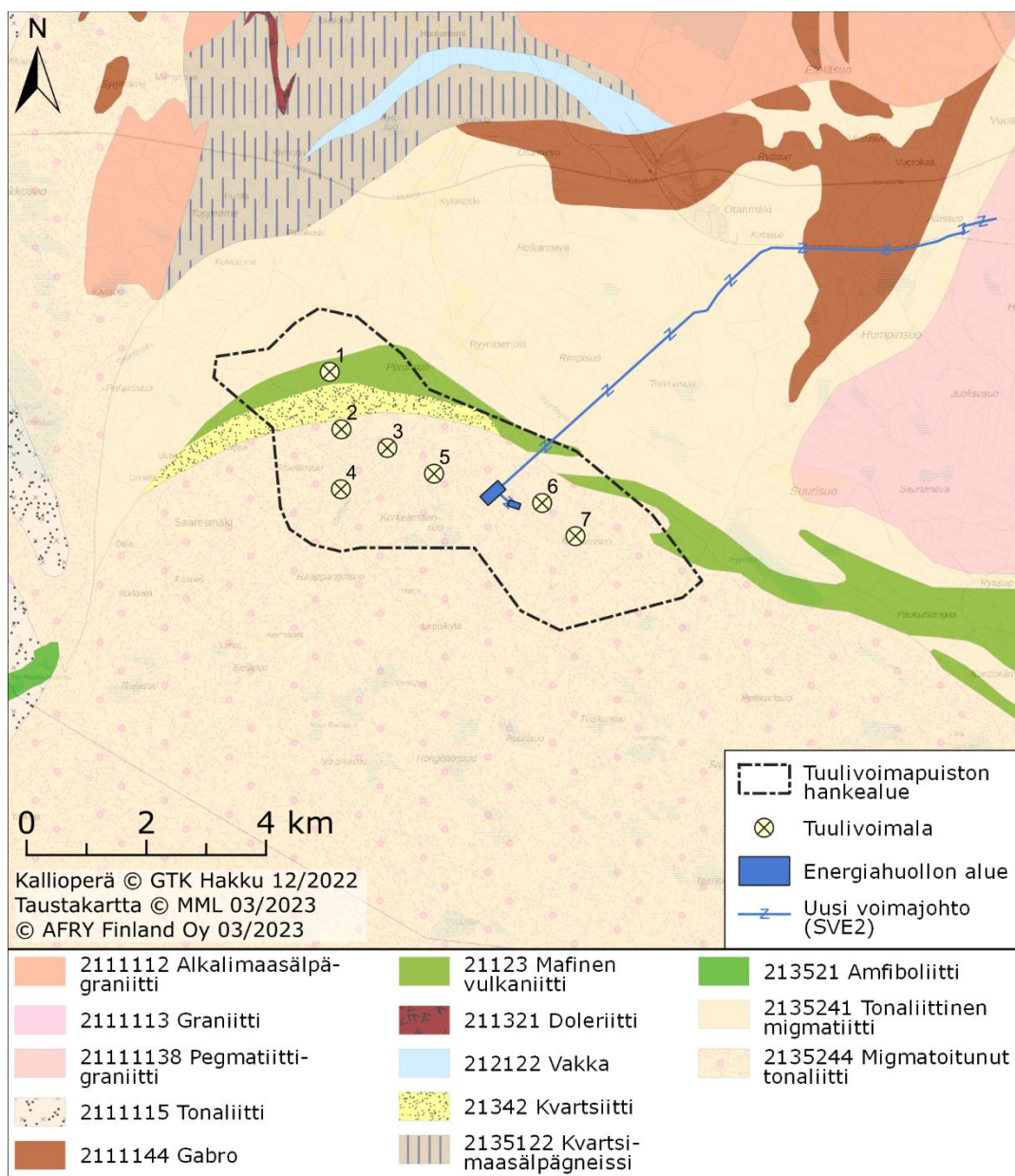
Kuva 5-17. Hankealueen kallioperä.
