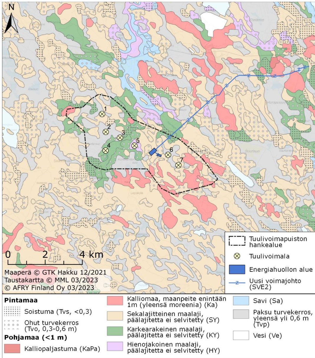
Kuva 5-16. Hankealueen maaperä.
